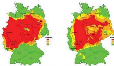
Extreme Bodenfeuchtesituation am 8. Juni 2015
